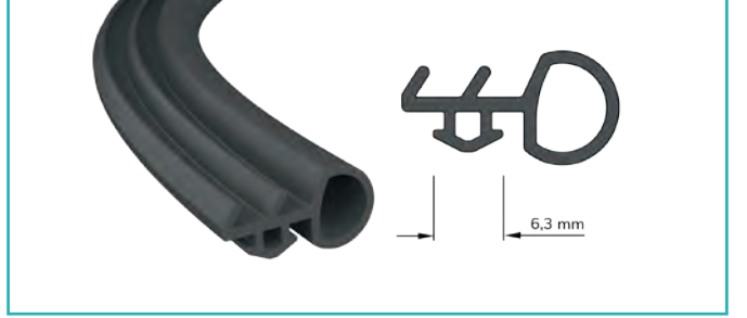
Vidasız Montaj Fitili Screwless Mounting Seal
