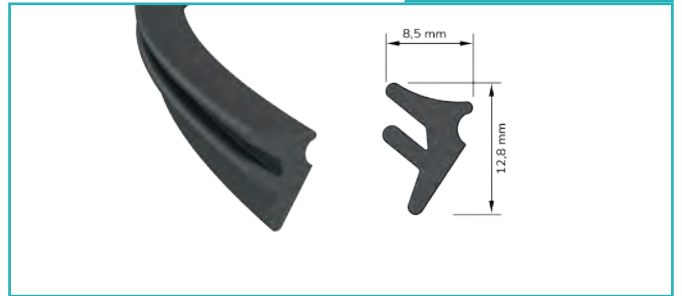
Tırnaklı Cam Contası Spiked Glass Joint
