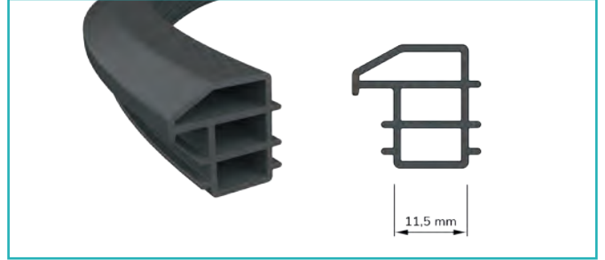
Çelik Kapı Fıtili Steel Door Seal
