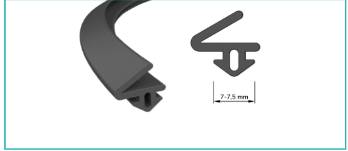
Yarıklı Conta 7-7,5 mm. Splint Joint 7-7,5 mm.
