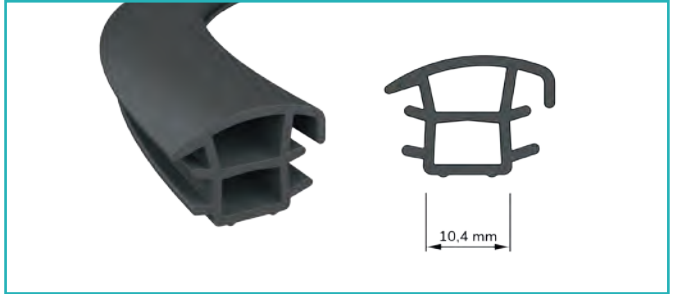
Çelik Kapı Fiteli Steel Door Seal
