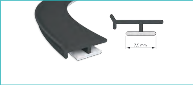
Sert Yumuşak Maçalı Fitol 7 mm. Hard Soft Cored Seal 7 mm.
