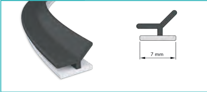
Sert Yumuşak Aldoks Çift kulak 7 mm. Hard Soft Aldoks Double Ear 7 mm.
