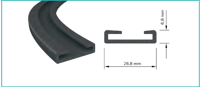
Sac Kenar Fiteli Sheet Metal Edge Seal
