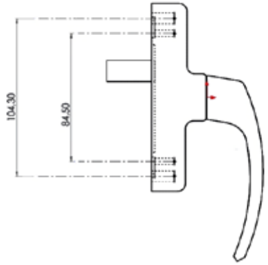
ISPANYOLET KOL CREMONE HANDLE
