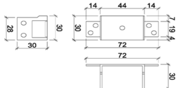
PVC ORTA KAYIT BAĞLANTI TAKOZU PVC STEEL MIDDLE JOINT مثبت بروفيلات ألمنيوم CODE : AB 012-F
