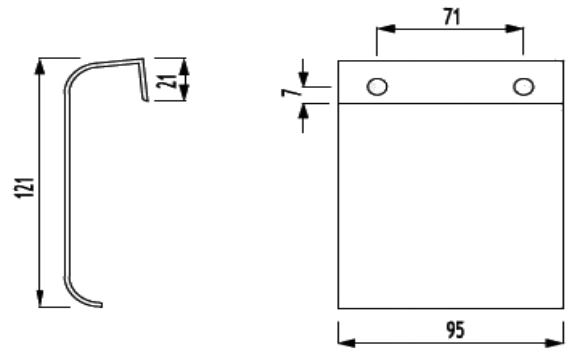
AKBANK YOL APARATI PULL HANDLE COMPLEMENT مسكة أبواب زجاج CODE : AB 172-D
