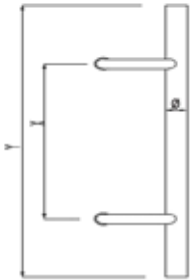
H KOL KÖŞELİ PULL HANDLE مسكة أبواب زجاج CODE : AB 172-EH
