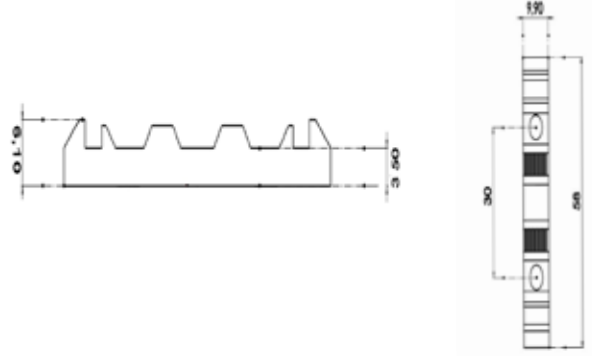
KELEBEK CEPHE KARŞILIĞI ADJUSTUBLE STRIKER 3
