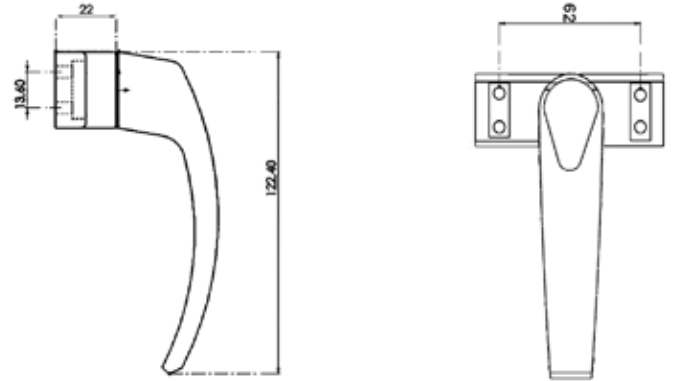
RAGNI YAYLI KAPI KOLU RAGNI DOOR HANDLE
