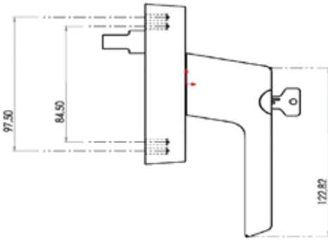
CEPHE KOL ZAMAK TEK MAÇA FACADE WINDOW HANDLE
