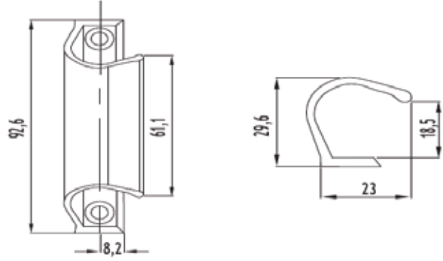
KARE KOL PULL HANDLE مسكة أبواب زجاج CODE : AB 172-Z
