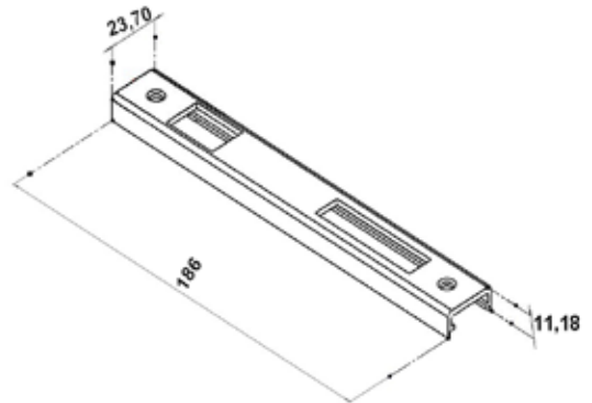
KAPI KİLİT KARŞILIĞI STRIKER FOR DOOR اكسسوارات أبواب CODE : AB 091-EK
