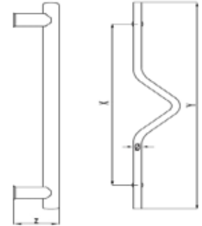
AYNALI BORU ÇEKME D KOL PULL HANDLE مسكة أبواب زجاج CODE : AB 172-0
