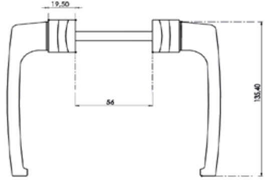
YAYLI KAPI KOLU 3 ALUMINIUM DOOR HANDLE
