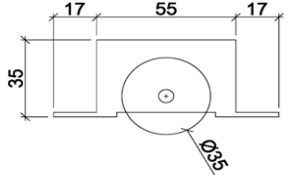
ÇİFT TEKER PİRİNÇ RULMAN
